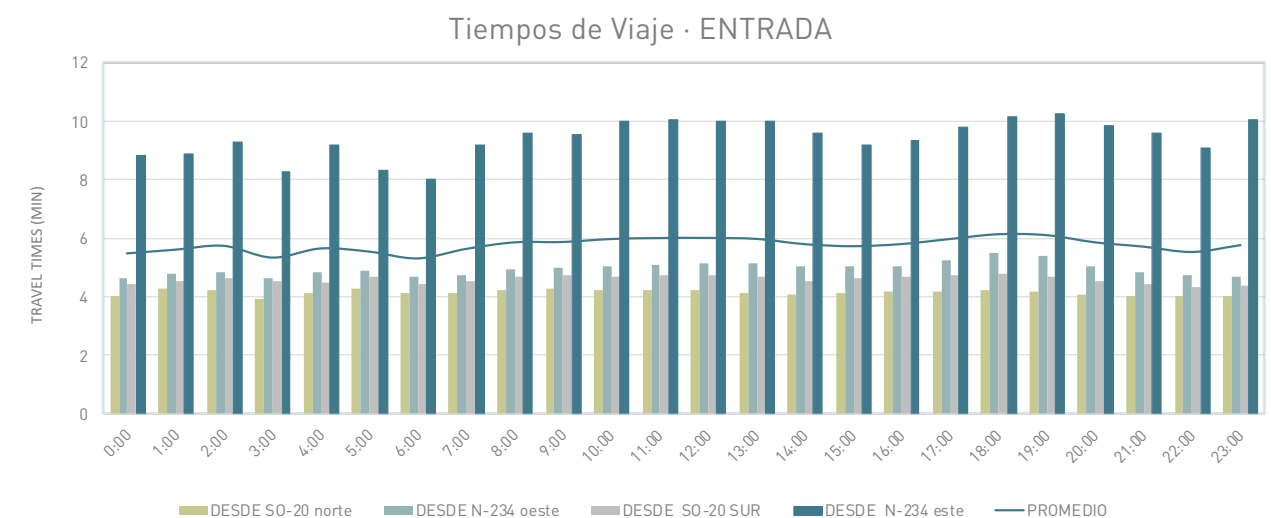
Imagen 19. Tiempos de viaje de entrada.
