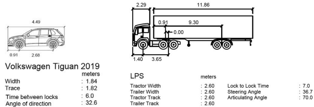
Imagen 45. Vehículos tipo utilizados.
