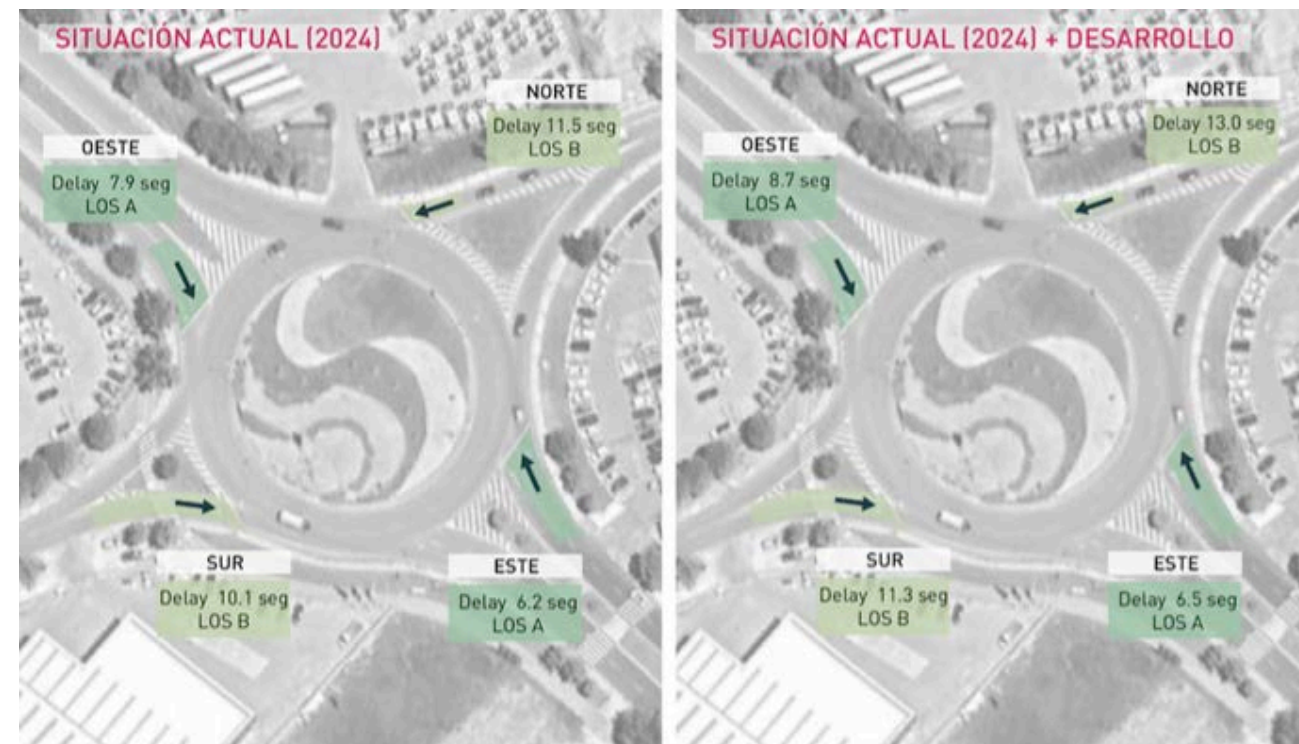
Imagen 51. Niveles de Servicio. P01 (2024).
