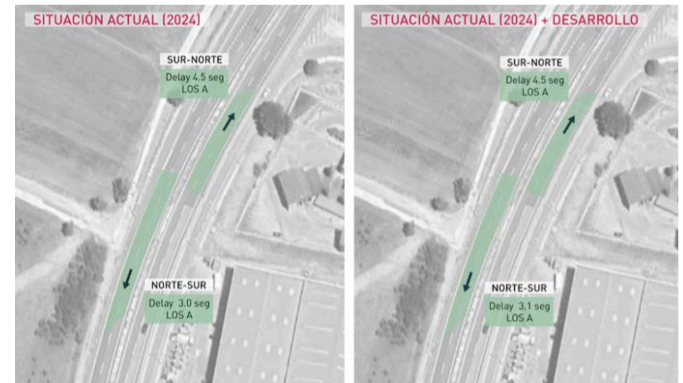
Imagen 55. Niveles de Servicio. Tronco SO-20 (2024).
