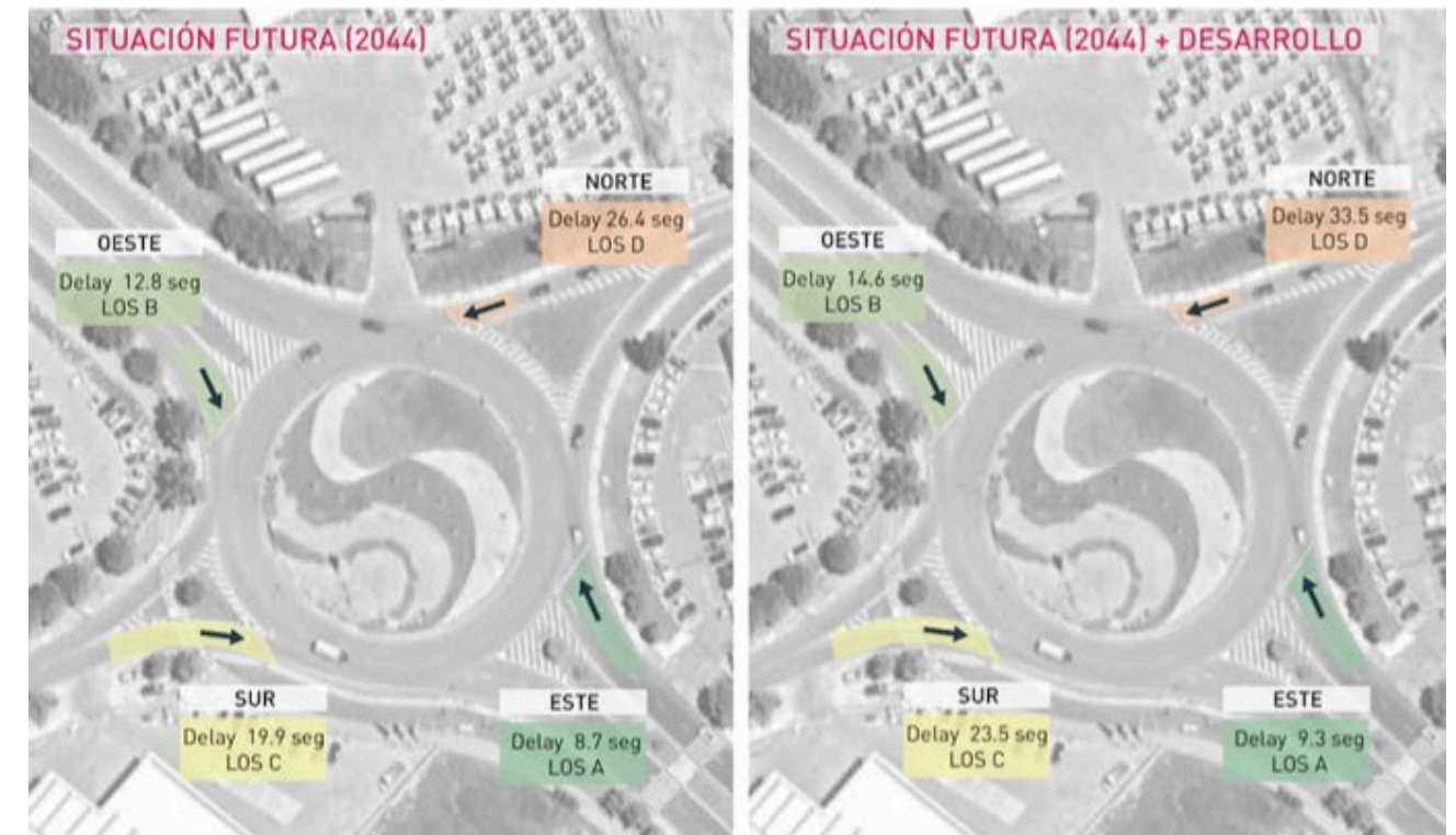
Imagen 52. Niveles de Servicio. P01 (2044).
