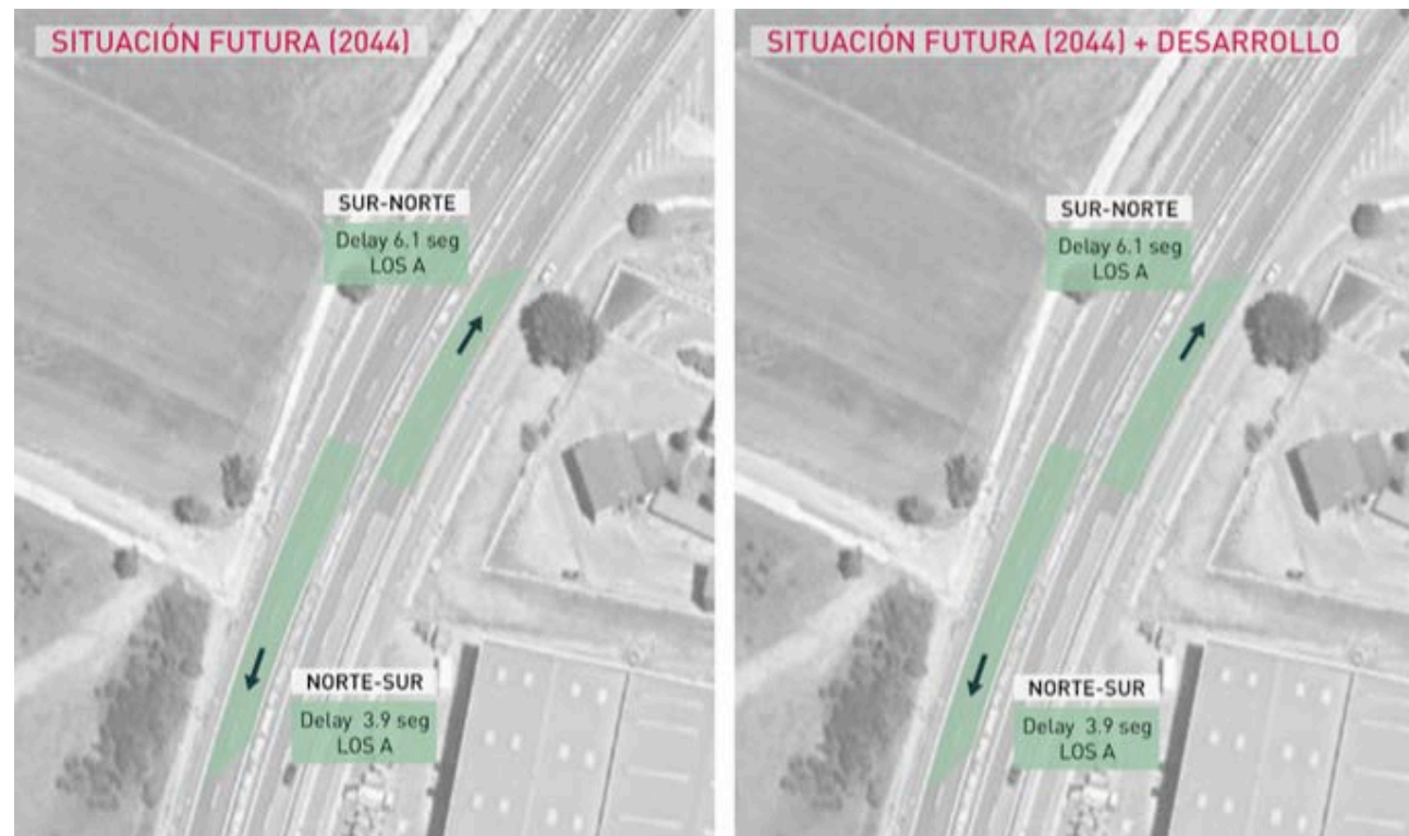
Imagen 56. Niveles de Servicio. Tronco SO-20 (2044).
