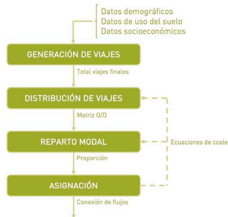
Imagen 42. Esquema del método de los cuatro pasos.
