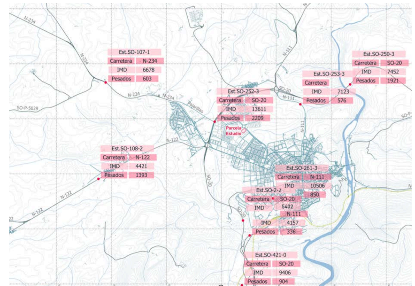
Imagen 22. Estaciones de aforo del entorno.
