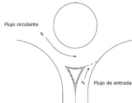
Imagen 50. Flujos de tráfico en una glorieta.
