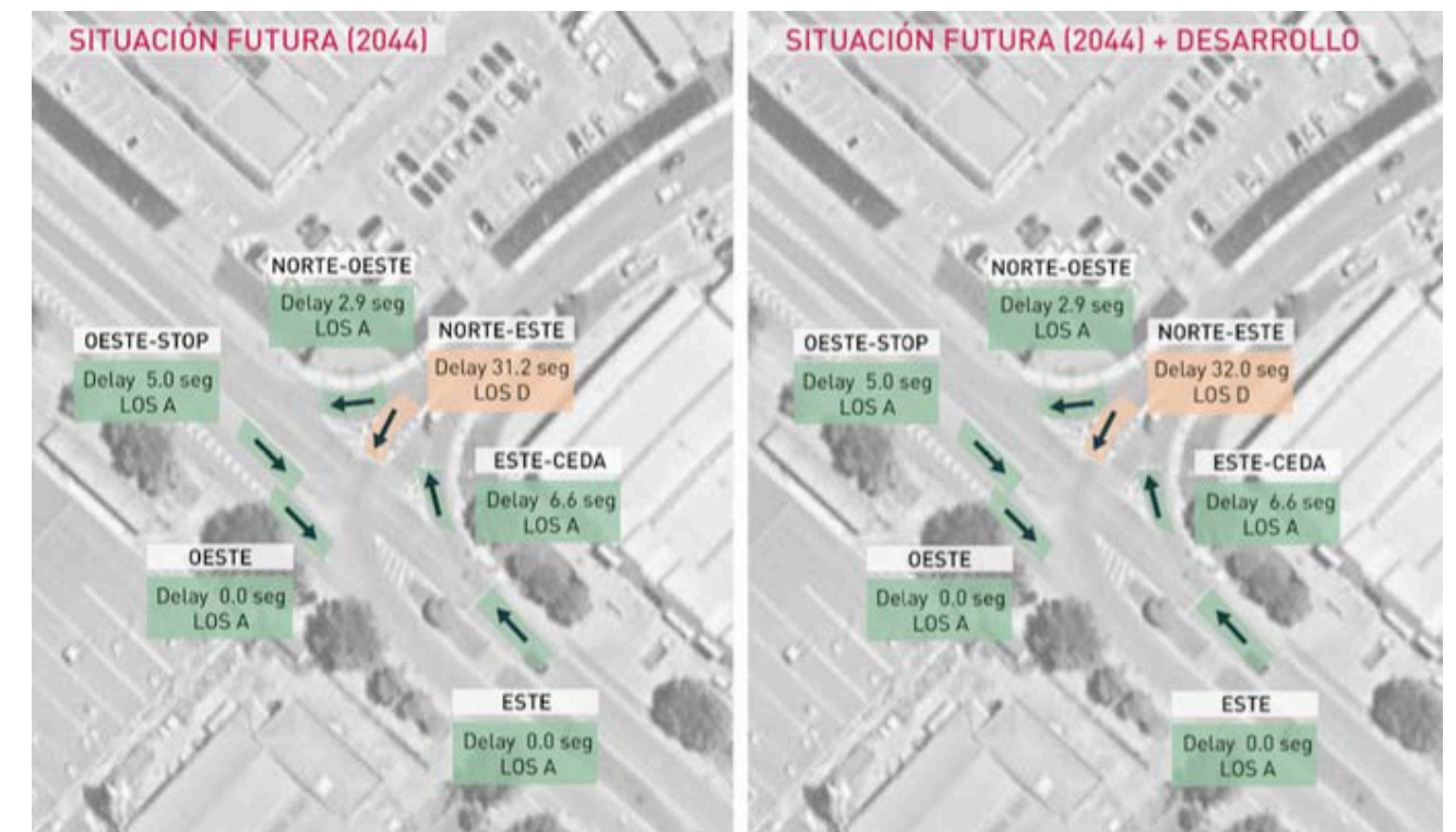
Imagen 54. Niveles de Servicio. P02 (2044).
