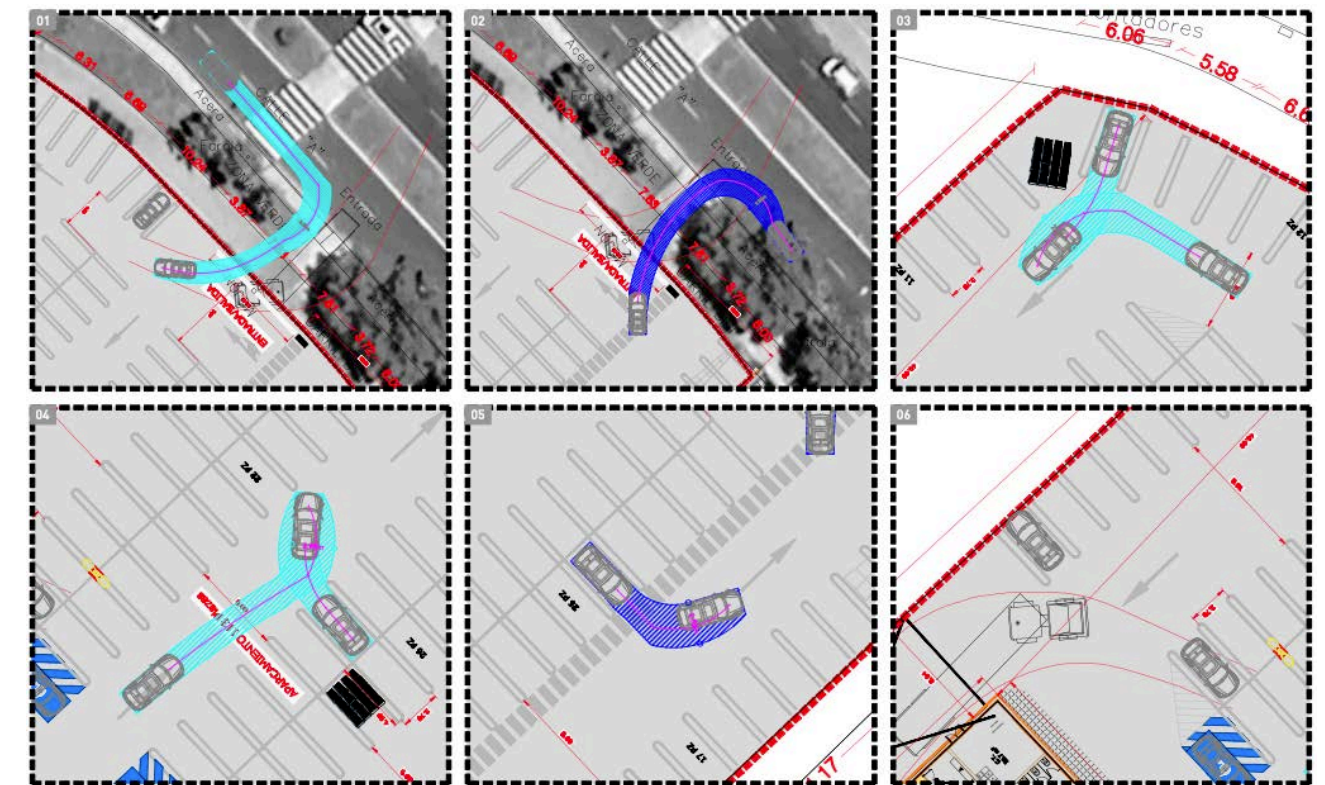
Imagen 46. Comprobación de giros de los vehículos ligeros.
