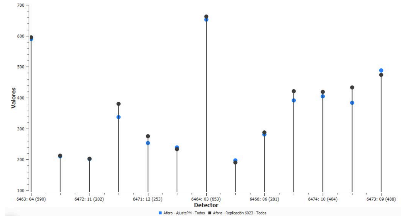
Imagen 26. Detalle Calibración del Modelo en PM.
